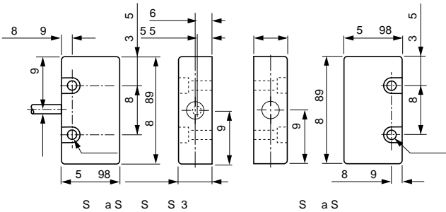
Sipha S1
