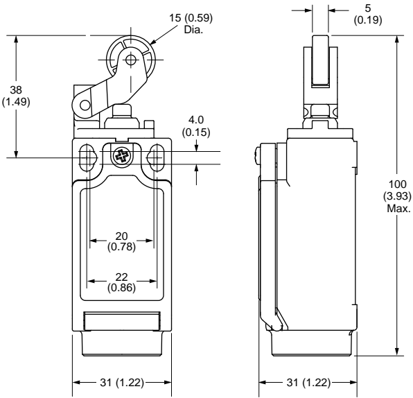
Hinge Lever
