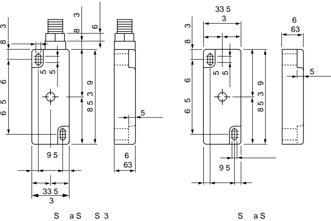
Sipha S4
