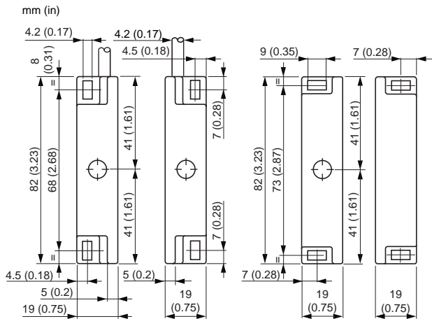
Sipha S2
