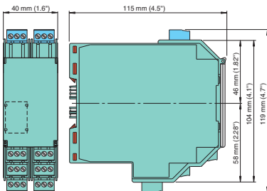
Maße des KF**-CRG2-(Ex)1.D in mm
