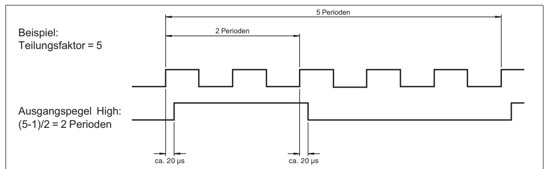
Abbildung 3.3 Teilungsfaktor 5
