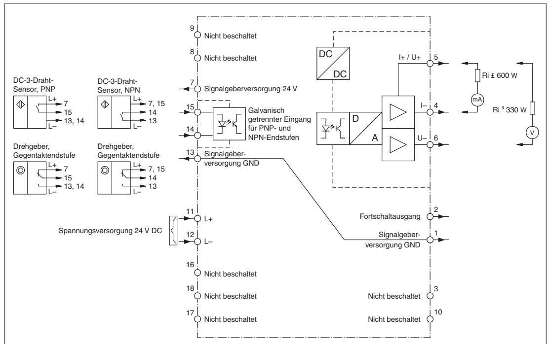
Abbildung 4.1 Anschlussplan
