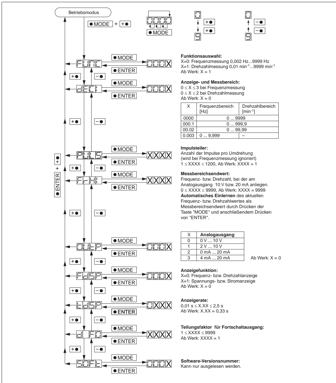
Abbildung 4.2 Grafische Funktionsbeschreibung
