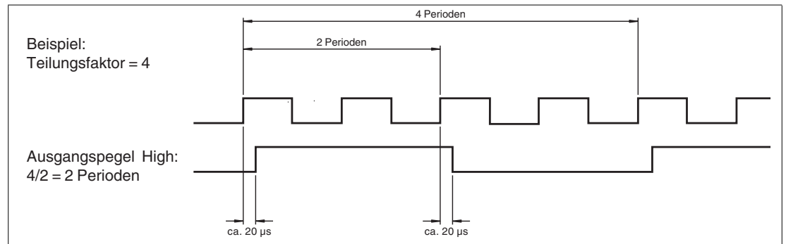
Abbildung 3.2 Teilungsfaktor 4
